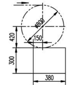
H1型清扫器安装孔尺寸
